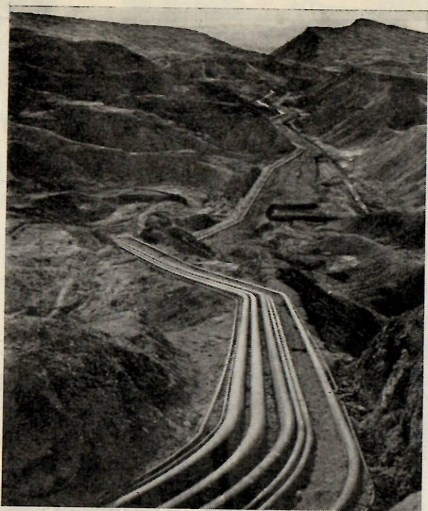
ΟΙ ΤΕΡΑΣΤΙΟΙ ΕΙΣ ΜΗΚΟΣ ΠΕΤΡΕΛΑΙΑΓΩΓΟΙ ΔΙΑΣΧΙΖΟΥΝ ΤΑΣ ΕΡΗΜΟΥΣ ΟΡΕΙΝΑΣ ΚΑΙ ΠΕΔΙΝΑΣ ΕΚΤΑΣΕΙΣ, ΔΙΑ ΝΑ ΜΕΤΑΦΕΡΟΥΝ ΤΟ ΠΕΤΡΕΛΑΙΟΝ ΕΙΣ ΤΟΥΣ ΛΙΜΕΝΑΣ ΤΟΥ ΠΕΡΣΙΚΟΥ ΚΟΛΠΟΥ ΚΑΙ ΤΗΣ ΑΝΑΤΟΛΙΚΗΣ ΜΕΣΟΓΕΙΟΥ.
